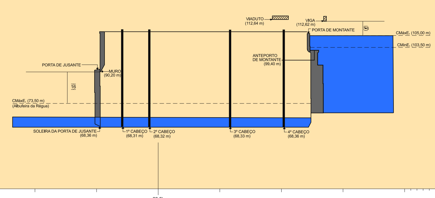
ESQUEMA VERTICAL DA ECLUSA DA BARRAGEM DA VALEIRA VERTICAL CROSS SECTION OF VALEIRA'S CANAL LOCK
